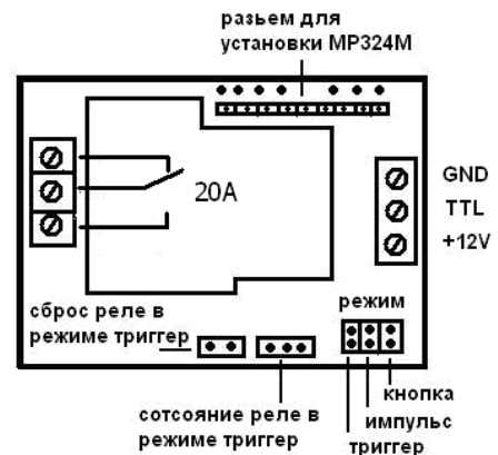
Схема подключения. Рис. 2
