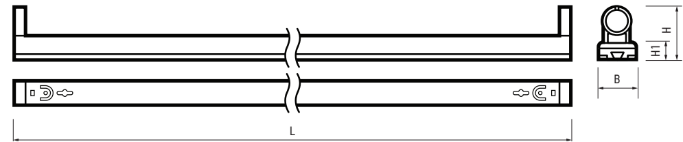
Рис.1 Светильник РРО-Т8
