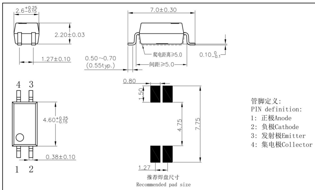
图 4 HPC214×h 外形尺寸 Figure 4- The dimensions of HPC214×h
