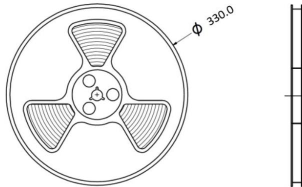
图 6 编带包装示意图
