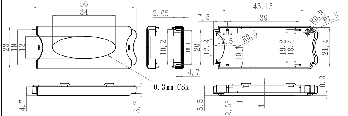
LID
