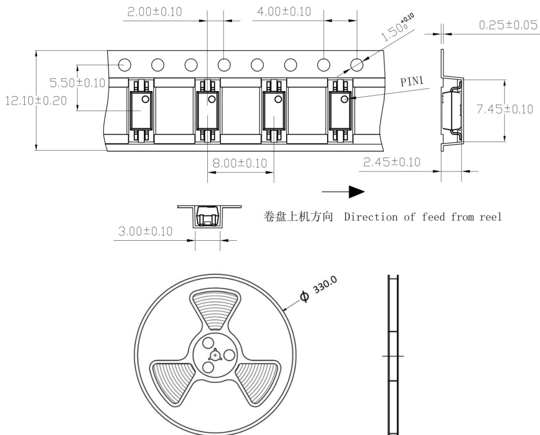
图 6 编带包装示意图
