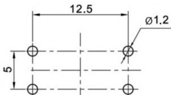
Макет (вид сверху)
