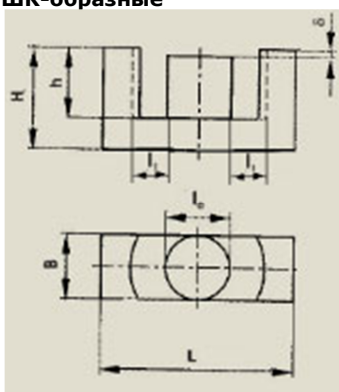
Размеры ШК- и Ш-образных сердечников.
