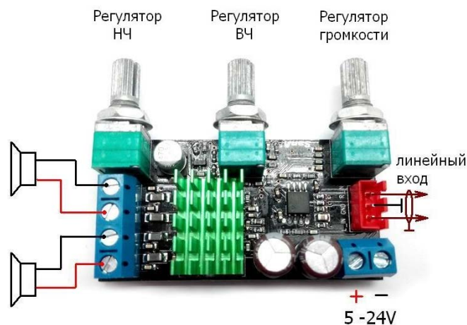
Эскиз подключения
