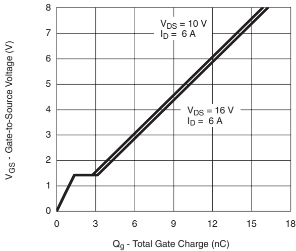
V_{DS} = 10 V I_D = 6 A V_{DS} = 16 V I_D = 6 A Gate Charge
