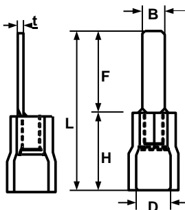
Сечение провода: 4-6мм 2 ; (A.W.G12-10) I max =48A Материал: медь. Толщина: 1,0мм
