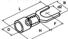
Сечение провода: 1,5-2,5мм 2 ; (A.W.G16-14) I max =27A Материал: медь. Толщина: 0,8мм
