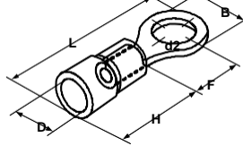
Сечение провода: 1,5-2,5мм 2 ; (A.W.G16-14) I max =27A Материал: медь. Толщина: 0,8мм
