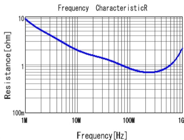
■ DE2B3SA471KA3BY02F R DCOV, 20degC
