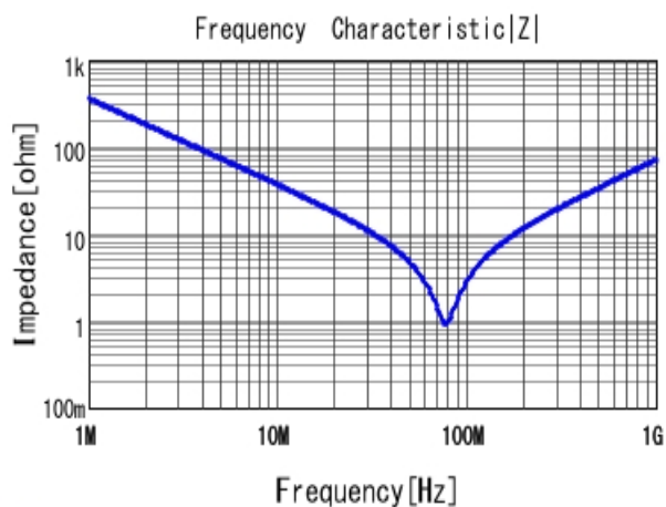
■ DE2B3SA471KA3BY02F |Z| DCOV, 20degC
