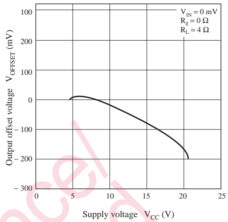
V_{OFFSET} - V_{CC}
