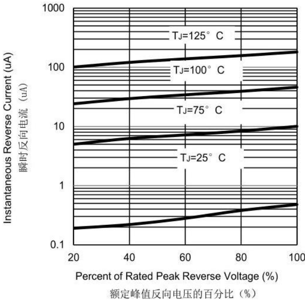
Fig. 3 - Typical Reverse Characteristics 图3 典型的反向特性
