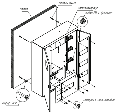
Рис. 1 - Схема монтажа
