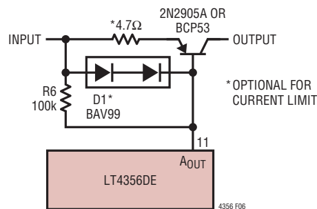
図6. オプションの電流制限付き補助LDO出力
