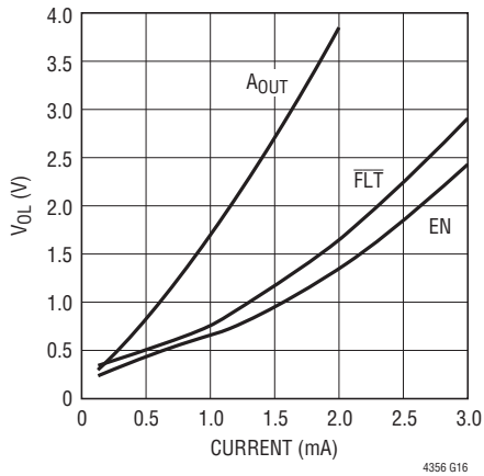
出力“L”電圧と電流
