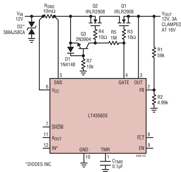
図7. NチャネルMOSFETの逆入力保護付き過電圧レギュレータ
