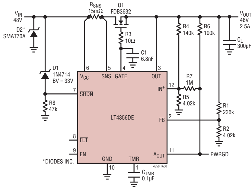
72Vでの過電圧出力レギュレーションと35VでのUVシャットダウン機能付きの2.5A、48Vホットスワップ
