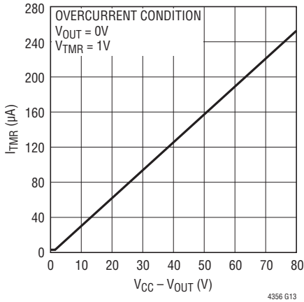
過電流TMR電流と (V_{CC}-V_{OUT})
