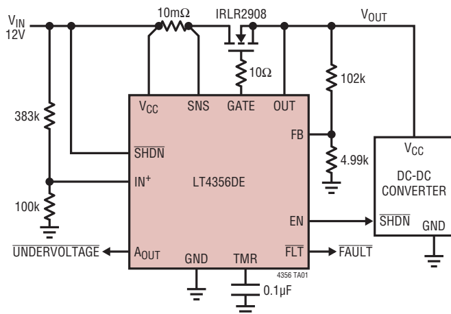
4A、12V過電圧出力レギュレータ
