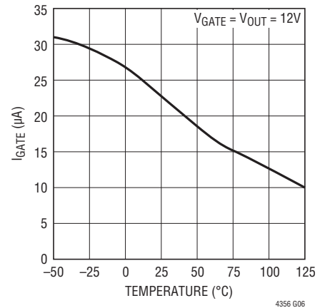
GATEプルアップ電流と温度
