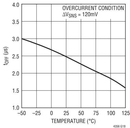
過電流ターンオフ時間と温度
