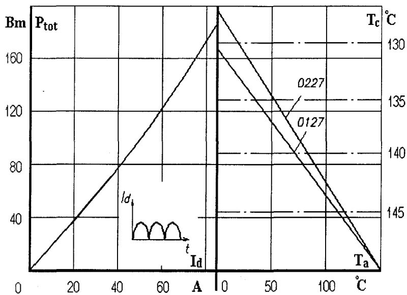
Рис. 2. 102.* Зависимости допустимой суммарной рассеиваемой мощности и допустимого выпрямленного тока двух модулей МДД4/3 - 80 на охладителях O127 и O227 от температуры окружающей среды и температуры корпуса при естественном охлаждении
