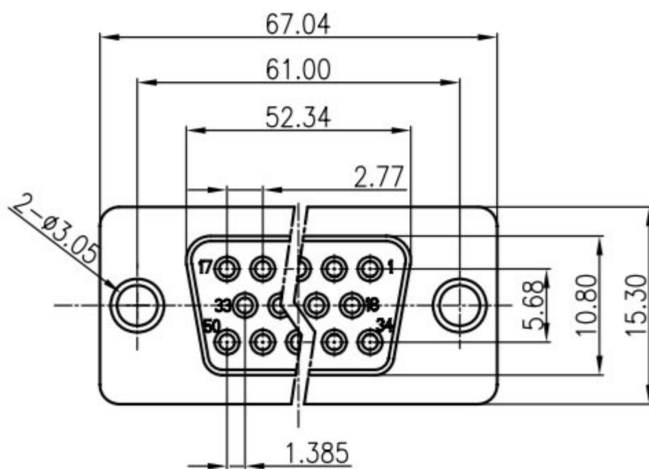
50-ти контактный разъем - розетка (F)
