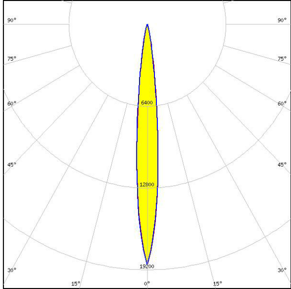
CREE XP-E
