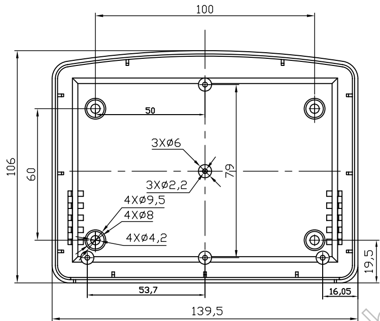
下盖主视图
