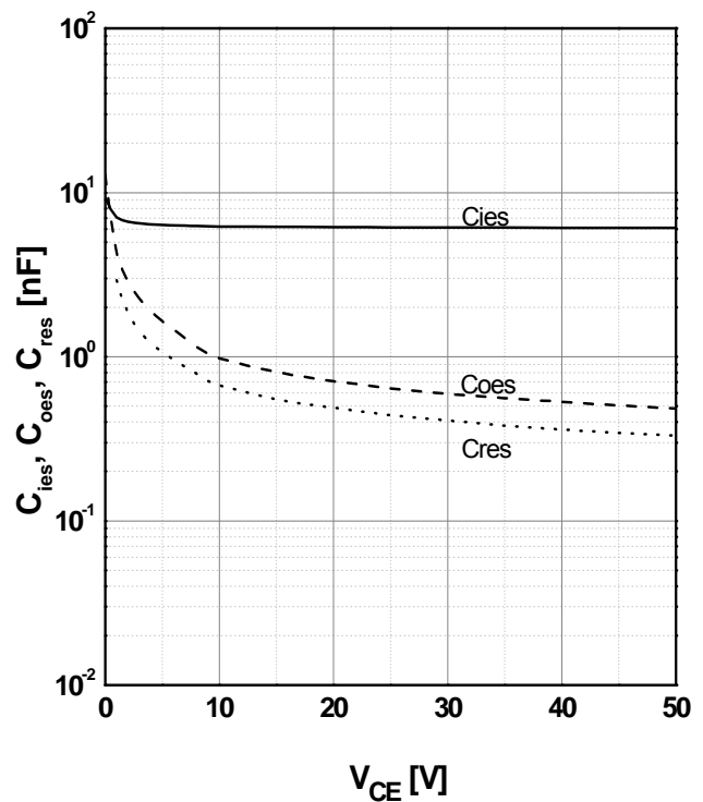
Fig8. Typ. Capacitance
