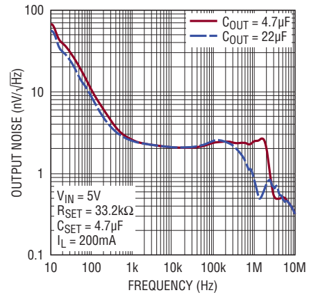
ノイズ・スペクトラム密度
