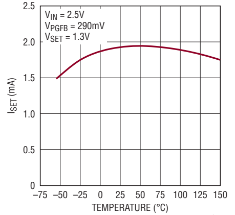
高速起動機能をイネーブルした場合の起動時の I_{SET}
