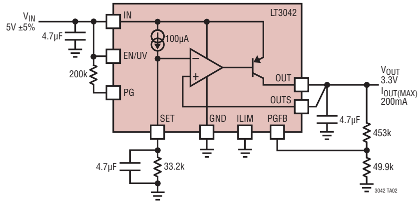
5V入力/3V出力、総合ノイズ:0.8 \mu Vrms
