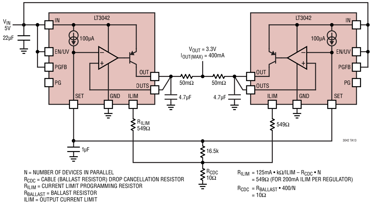
ILIM (電流モニタ)を使用した複数のデバイスの並列接続により安定抵抗での電圧降下を相殺
