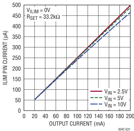
ILIM ピンの電流
