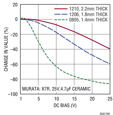
図6. 異なるケース・サイズでのコンデンサの電圧係数
