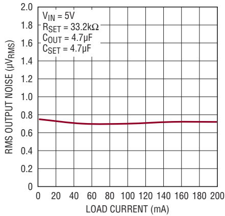
総合RMS出力ノイズ (10Hz~100kHz)
