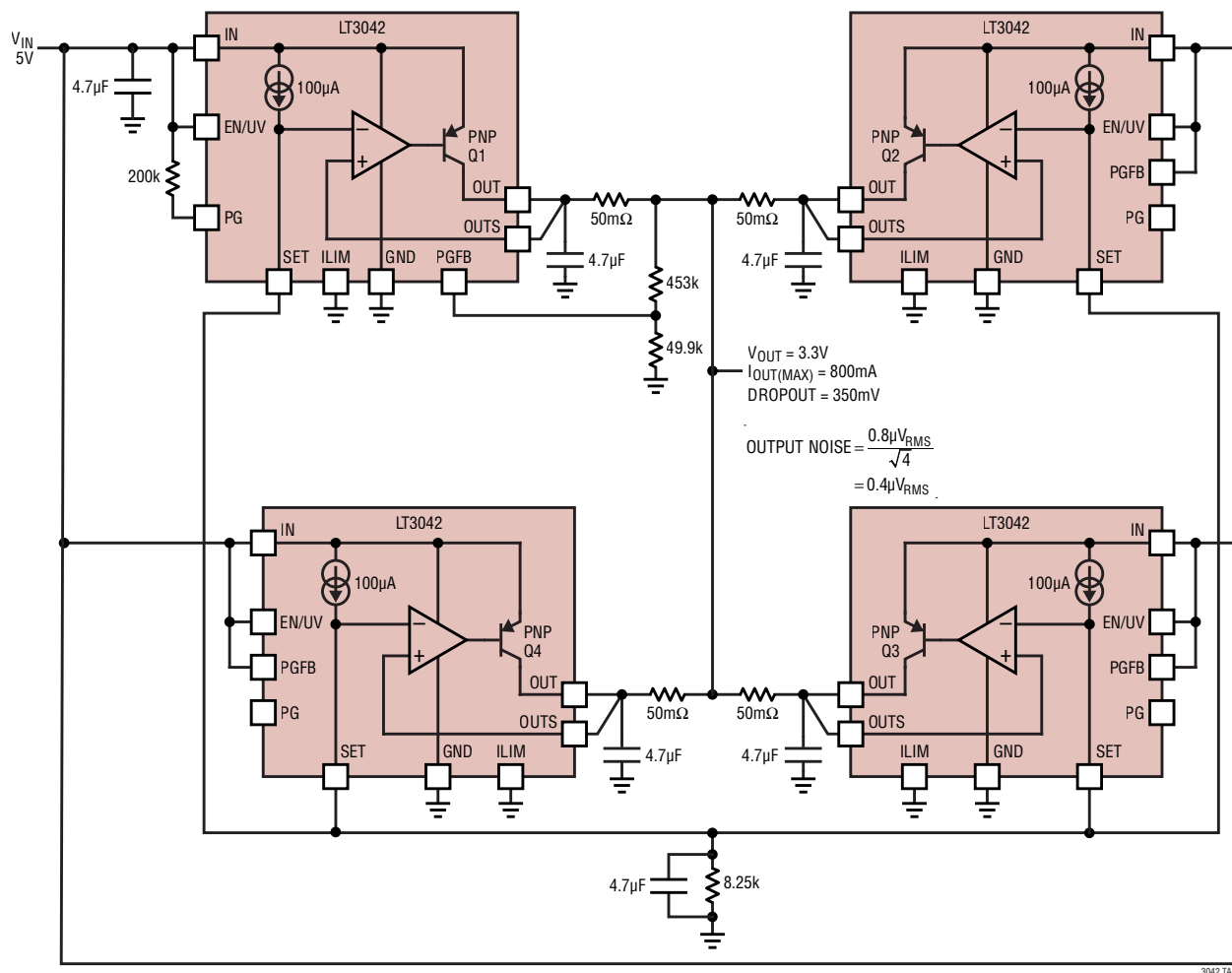
複数のLT3042の並列接続による大出力電流化
