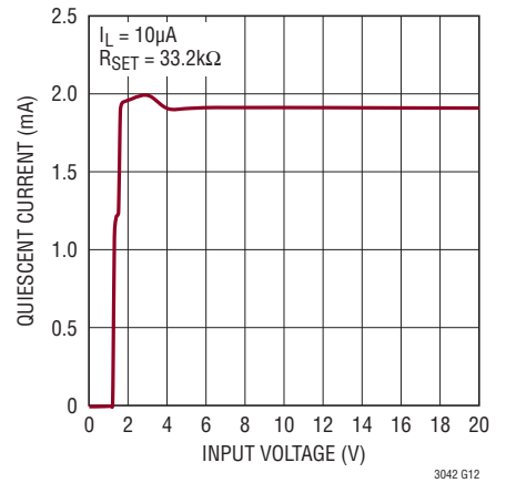
静止電流
