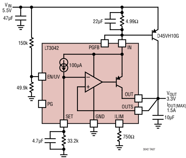
PNPを外付けした超低ノイズ大電流レギュレータ
