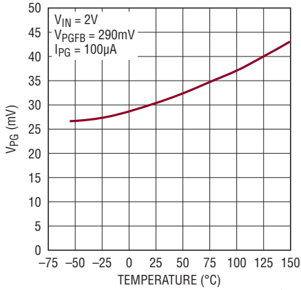
PG 出力の“L”電圧
