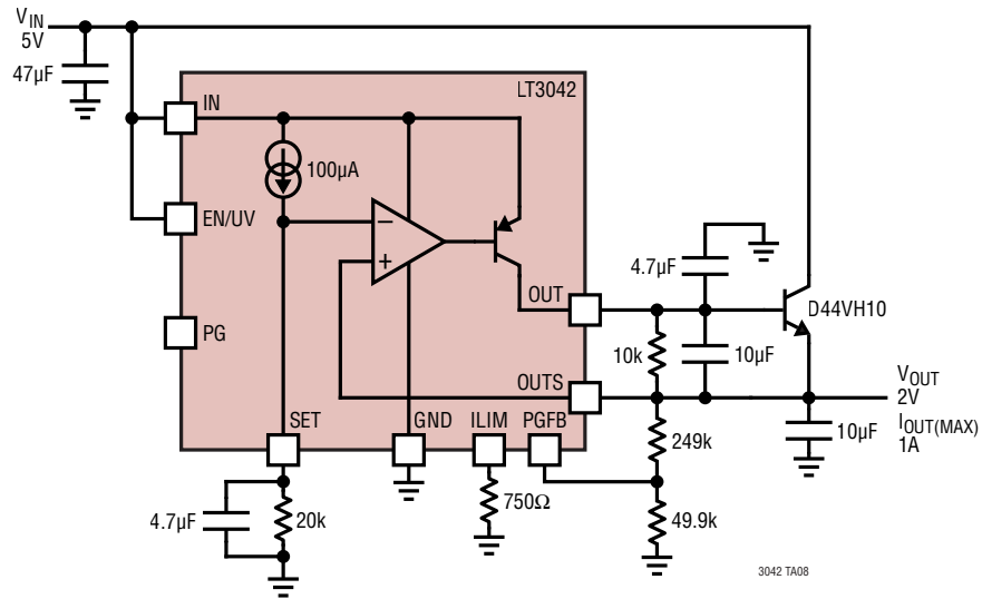
NPNを外付けした超低ノイズ大電流レギュレータ
