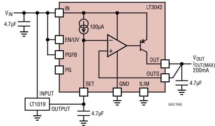
リファレンス・バッファ
