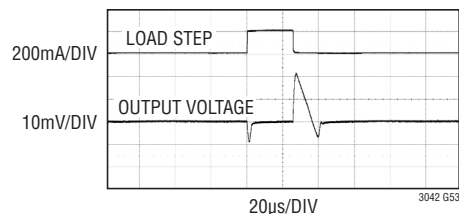
負荷トランジェント応答
