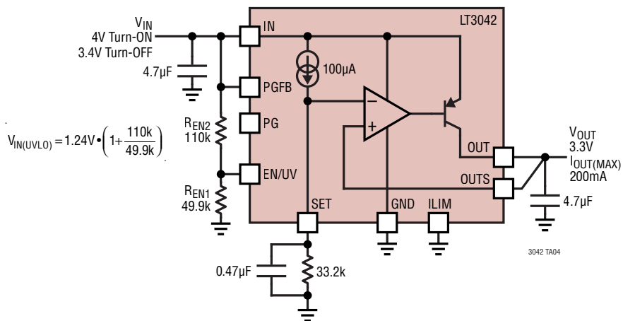
低電圧ロックアウトの設定
