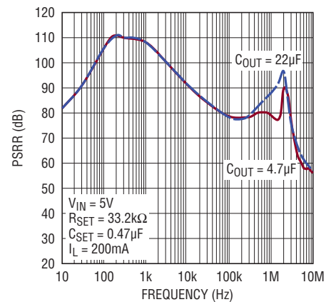
電源リップル除去比
