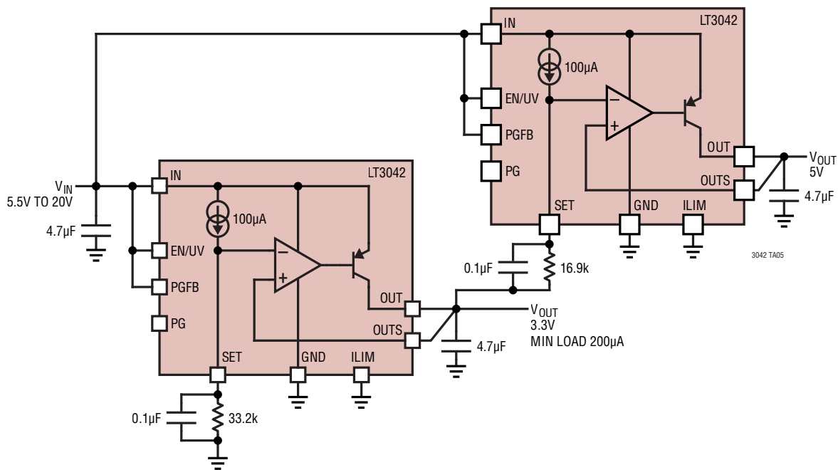
比例トラッキング
