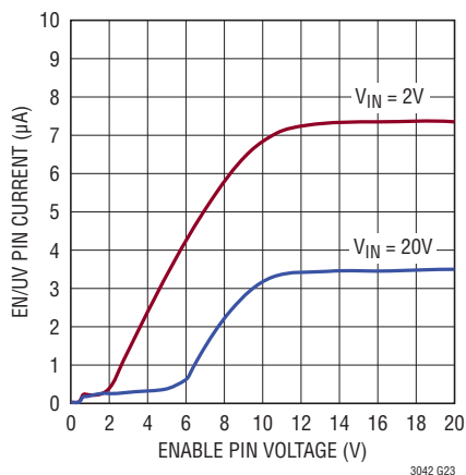
イネーブル・ピンの電流
