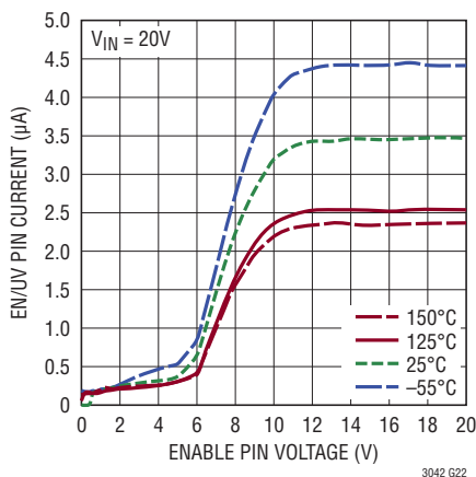
イネーブル・ピンの入力電流
