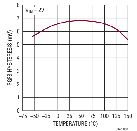
PGFB のヒステリシス
