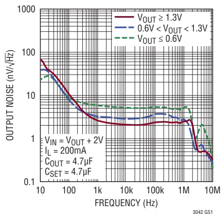
エラーアンプ入力対の関数としての ノイズ・スペクトラム密度
