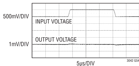
入力トランジェント応答
