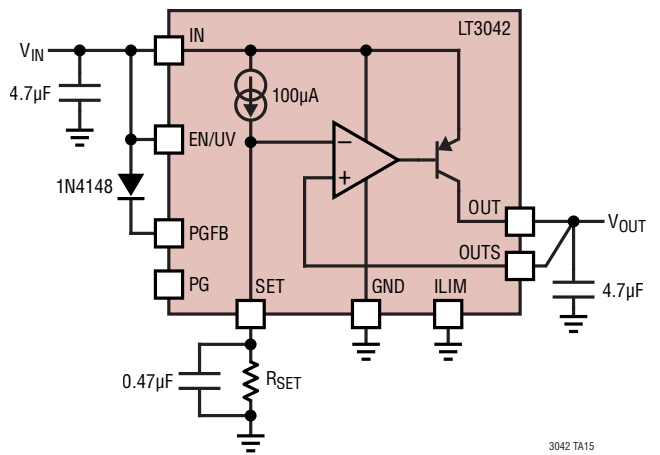
逆入力保護ありでPGFBをディスエーブル
