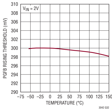
PGFB の上昇しきい値
