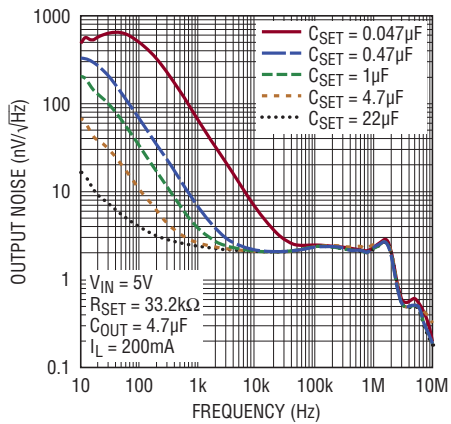
ノイズ・スペクトラム密度
