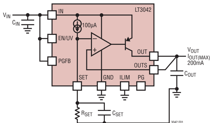
図3. C_{OUT} と C_{SET} の接続による安定性の確保
