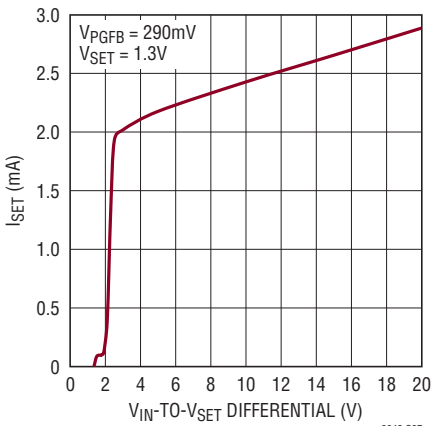
高速起動機能をイネーブルした場合の起動時の I_{SET}
