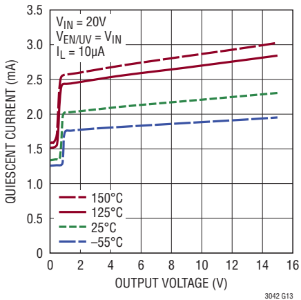
静止電流
