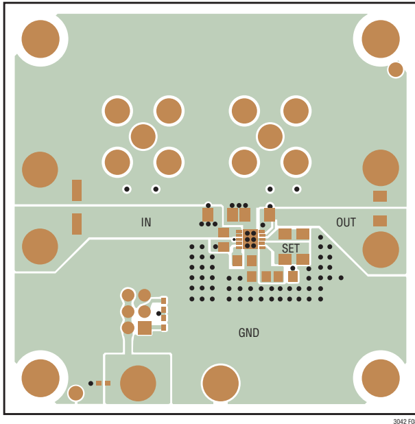
図 8. DFN レイアウトの例
