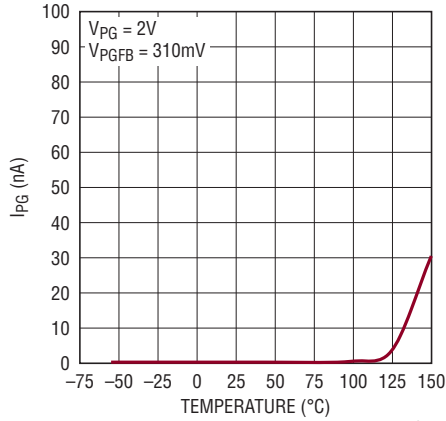
PG ピンの漏れ電流
