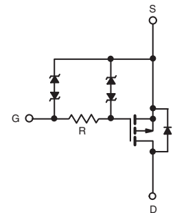
P-Channel MOSFET
