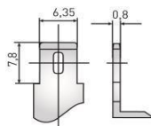
Клеммы нож F2
