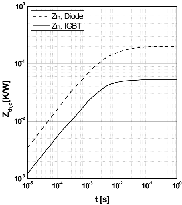
Fig7. Transient Thermal
