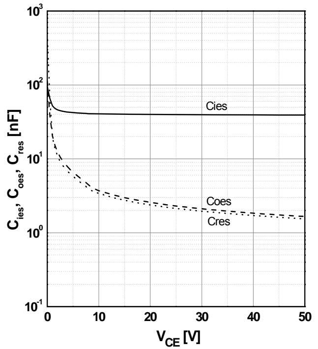
Fig8. Typ. Capacitance
