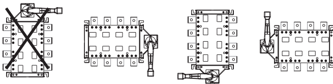
Рисунок 7 - Рабочее положение рубильников при эксплуатации
