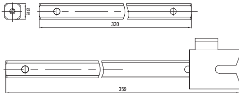
Рисунок 5 - Габаритные размеры штока
