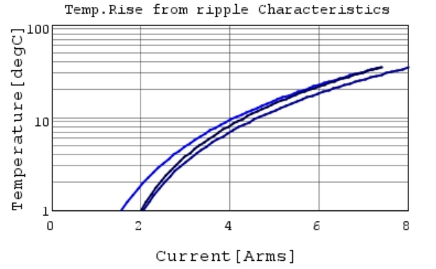
GRM32EC70J107ME15 Temp.rise — 50kHz
