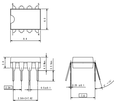
DIP-8
