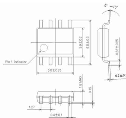
SO-8
