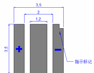
仰视图
