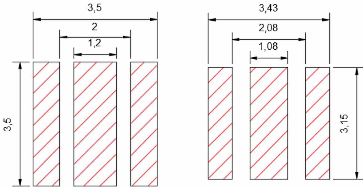
焊盘设计外形尺寸 (单位: mm)
