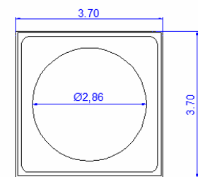
俯视图
