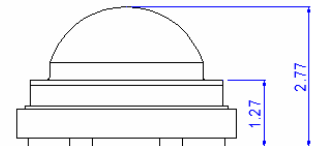
侧视图
