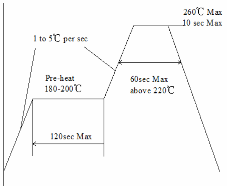
回流焊条件（无铅高温锡膏）
