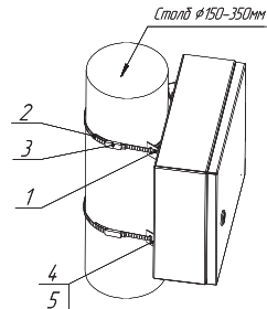
Рис. 1.2. Схема монтажа на столб (доп. аксессуар арт. mb54-1К)
